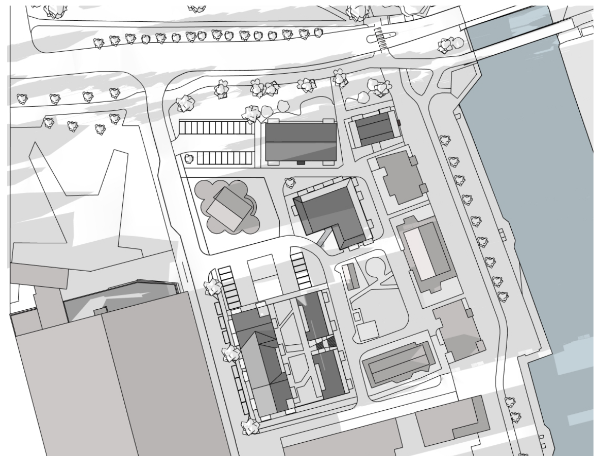
Vårdagjämning kl 17.00
