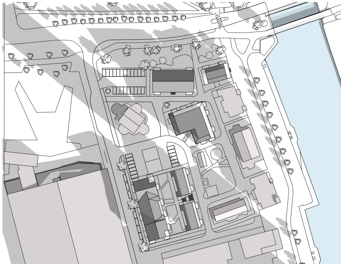
Vårdagjämning kl 09.00
