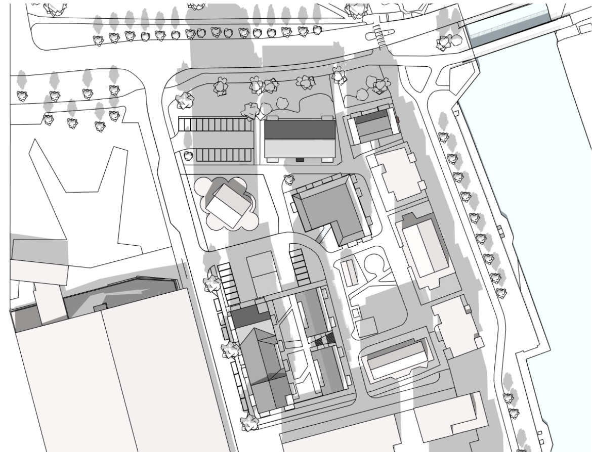
Vårdagjämning kl 12.00
