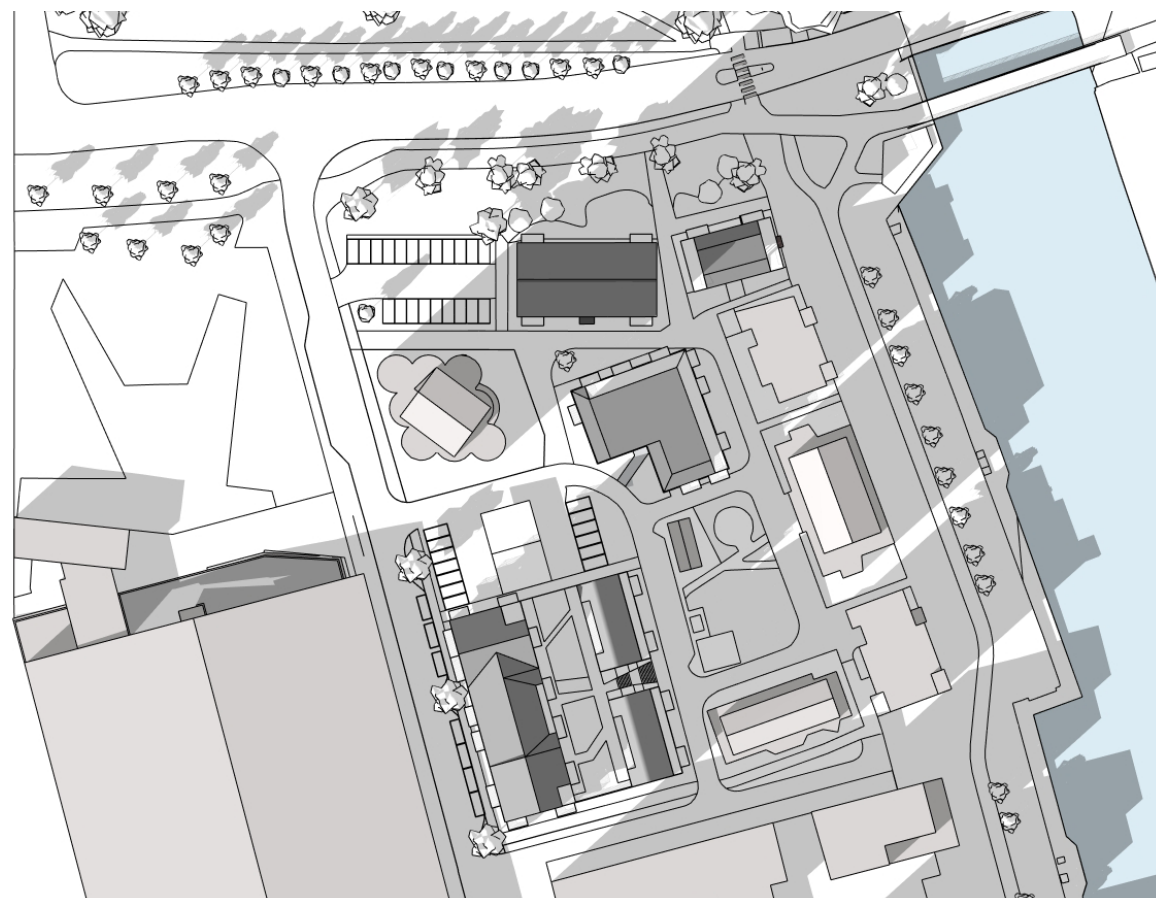
Vårdagjämning kl 15.00
