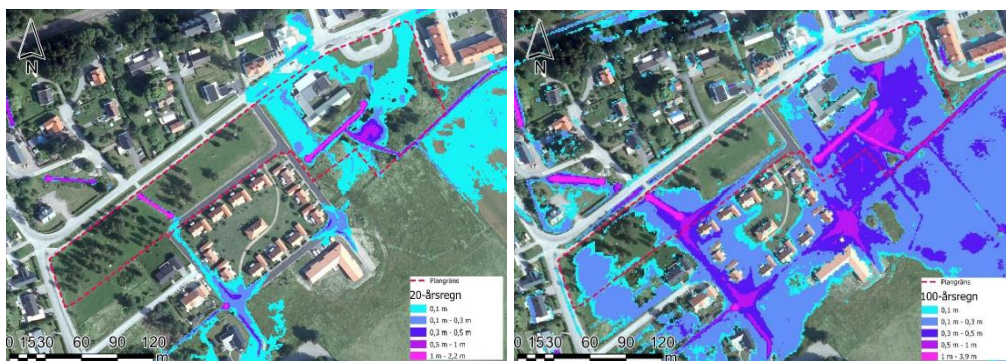
Figur 20. Kartbilder som visar maximal översvämning vid 20- respektive 100-årsregn i nulägesmodellen.
