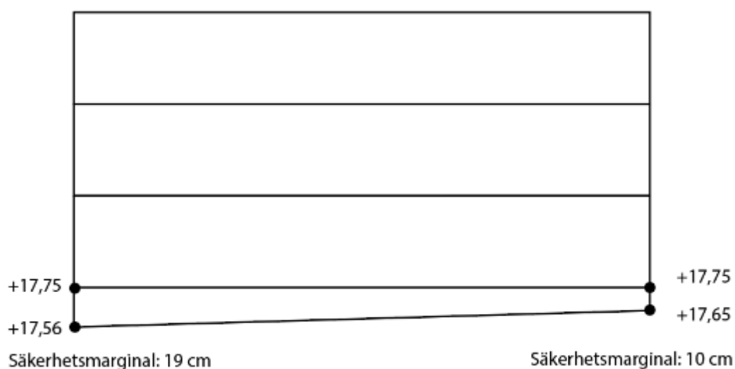
Figur 33. Principskiss som visar på hur nivån på färdigt golv regleras för att ligga med korrekt säkerhetsmarginal.
