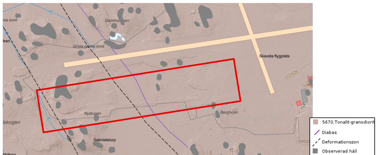
Figur 4. Berggrundskarta (©SGU). Utredningsområdet ungefärligt markerat i rött.
