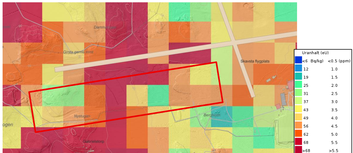
Figur 3. Gammastrålning från uran (©SGU). Utredningsområdet ungefärligt markerat i rött.
