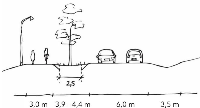
Figur 33. Gatusektion som visar utformningsexempel av entrégata in till området, vid infartens trädallé.
