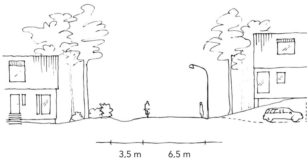
Figur 34. Gatusektion som visar utformningsexempel av kvartersgata inom området, inom delområde Skogen.
