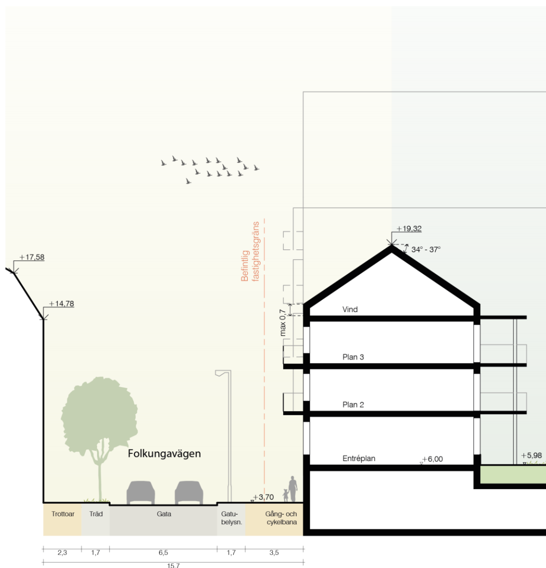
Figur 18: Gatusektion för Folkungavägen.
