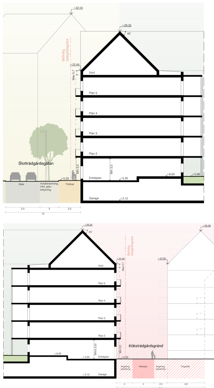
Figur 20: Sektioner för Slottsträdgårdsgatan och Köksträdgårdsgränd
