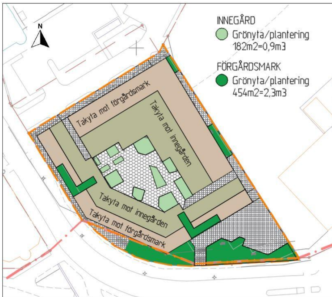
Figur 16: Dagvattenhantering.
