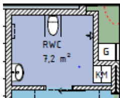
Exempel på toalett, badrum med dusch. Plats finns för överflyttning mellan rullstol och lös duschstol. 150 cm vänddiameter för rullstol uppfylls (SIS).
